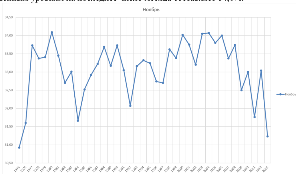
Рис. 9 Значения уровней Цимлянского водохранилища за ноябрь, 1975-2015 гг. в м БС
