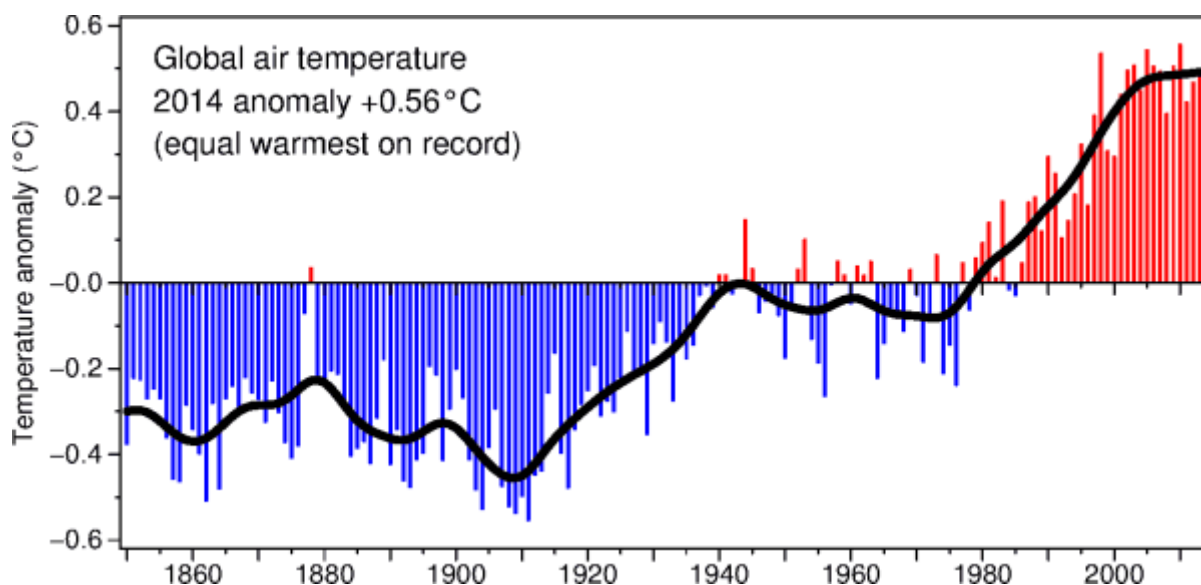
Рис. 2. Аномальный рост температуры за последние 120 лет (по данным Японского метеорологического агентства (JMA))
