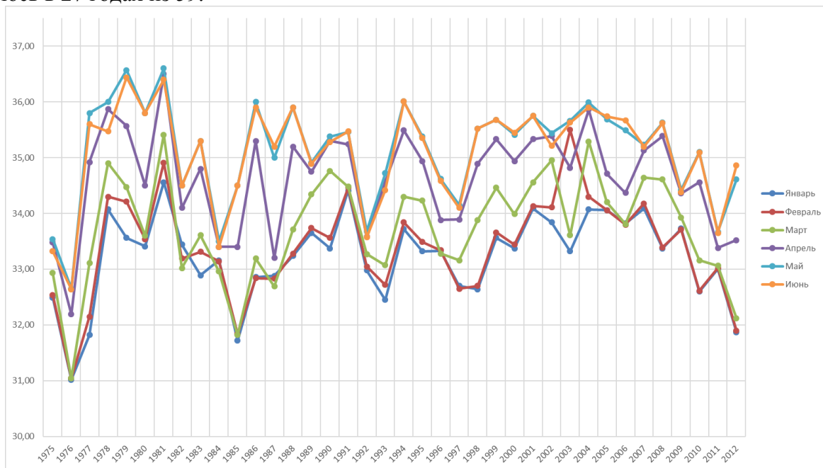
Рис. 7 Максимальные уровни Цимлянского водохранилища за январь-июнь, 1975-2012 гг. в м БС
