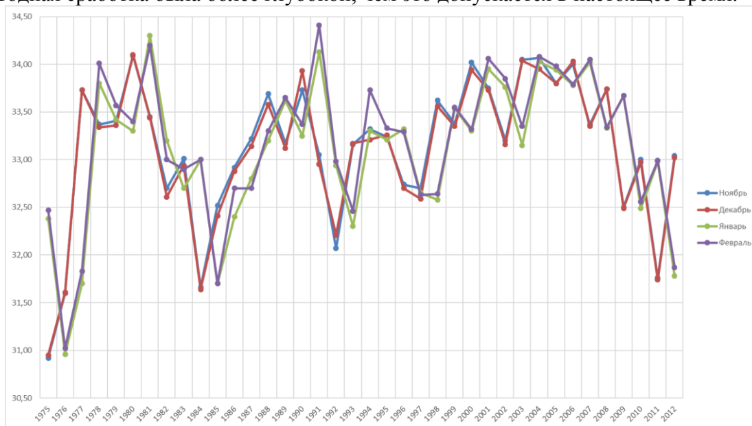
Рис. 8 Минимальные уровни Цимлянского водохранилища за ноябрь-февраль, 1975-2012 гг. в м БС
